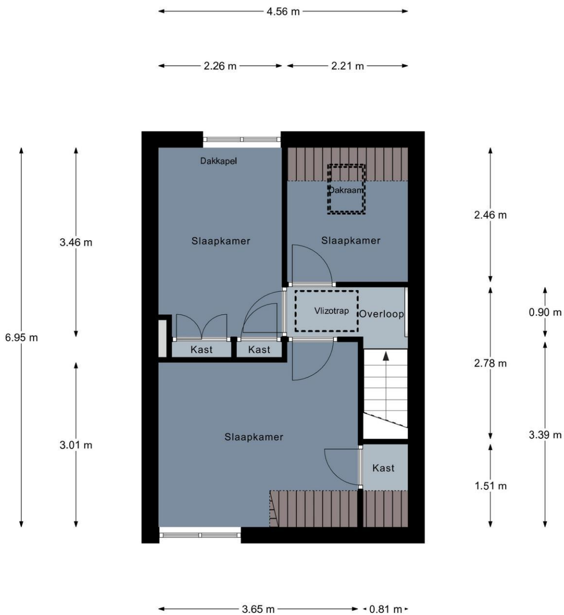
1e Verdieping
