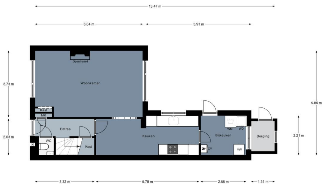
Begane Grond
