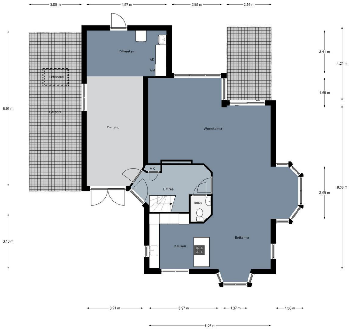
Begane Grond
