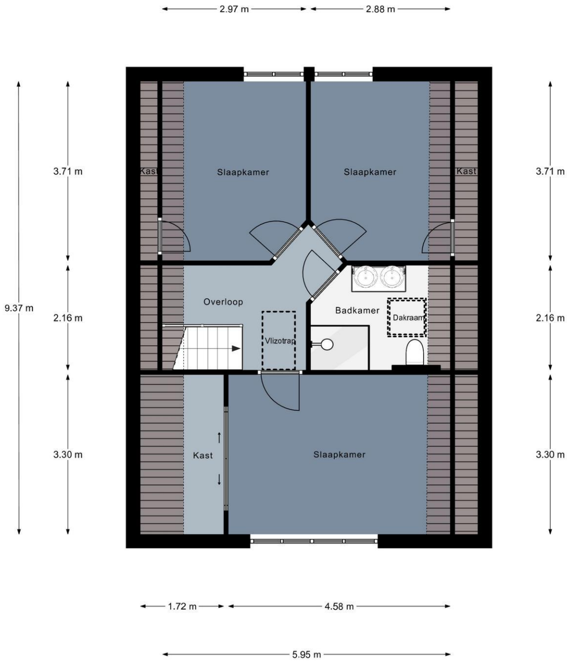
Eerste Verdieping
