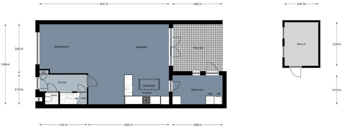
Begane Grond
