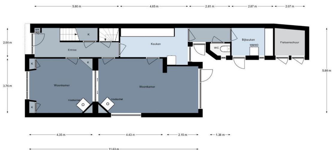
Begane Grond
